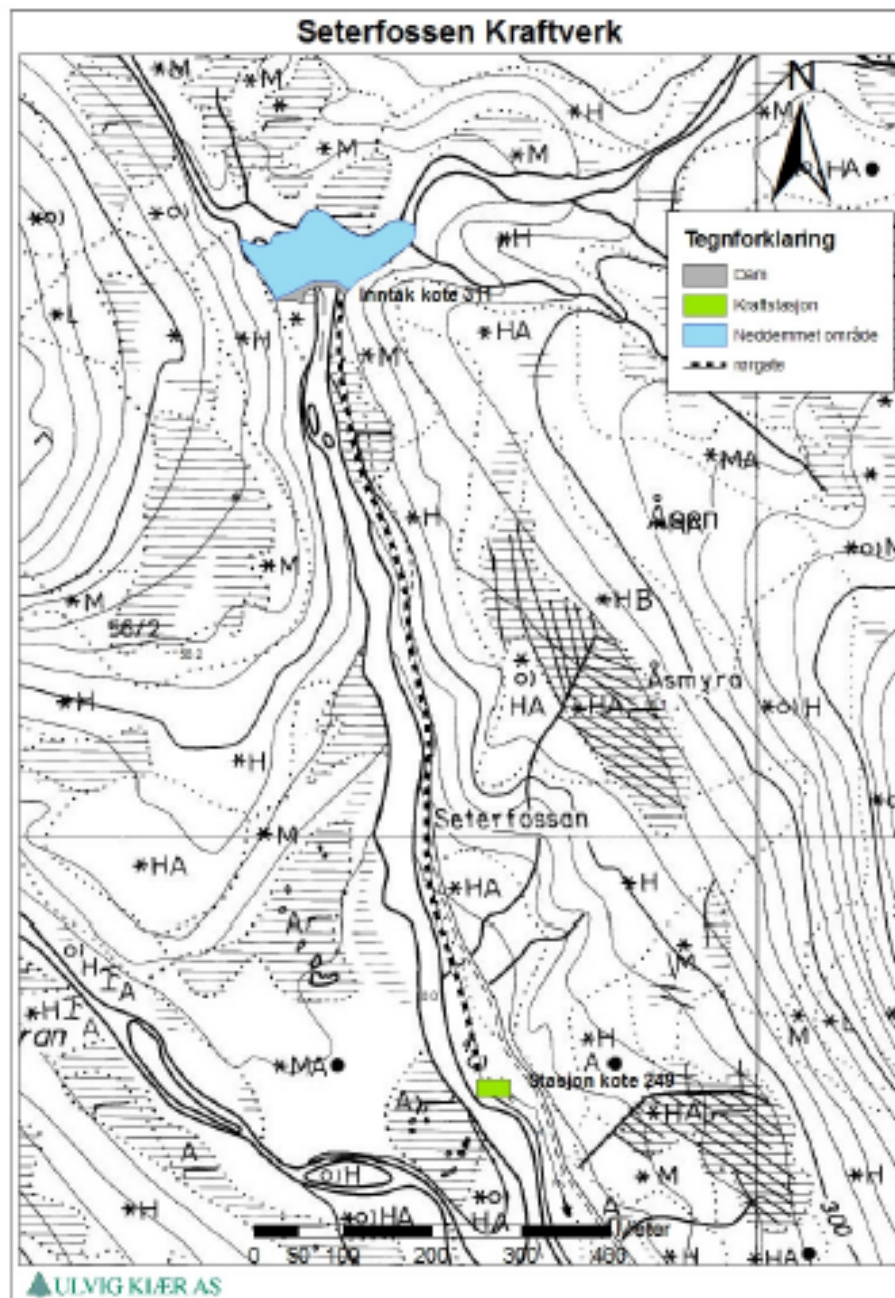
Vedlegg 2: Oversikt over anleggsdelene inntegnet på kart i målestokk 1:5000. (Se målestokk inntegnet)
